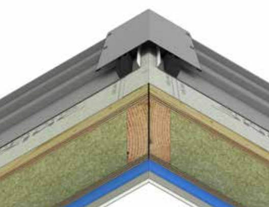
faîtage G3 - toiture non aérée nok G3 niet verlucht dak
