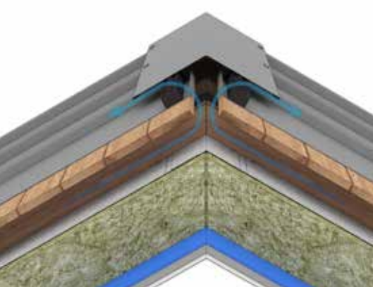
faîtage G3 - toiture aérée nok G3 verlucht dak
