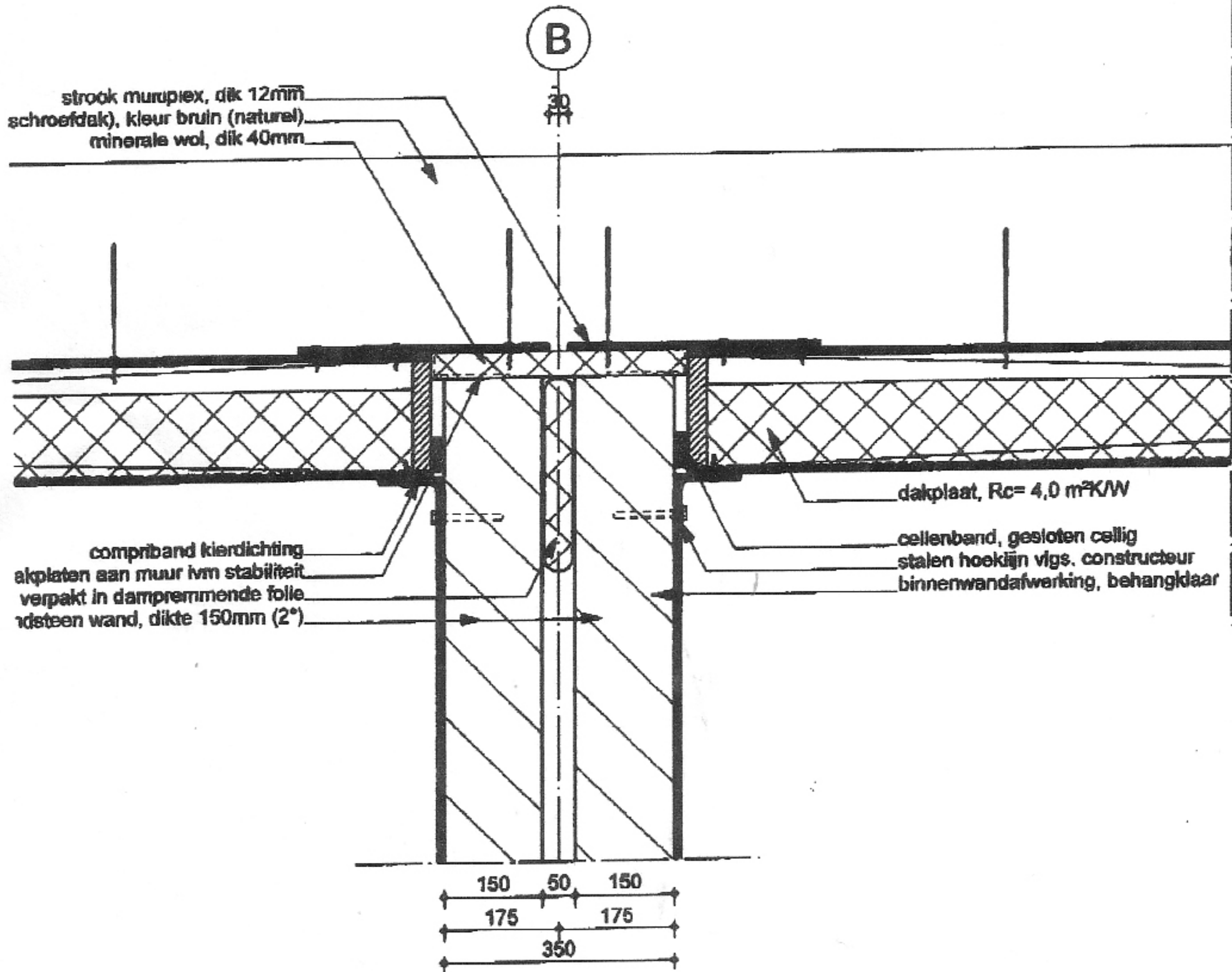
Dak t.p.v. woningscheidende wand.
