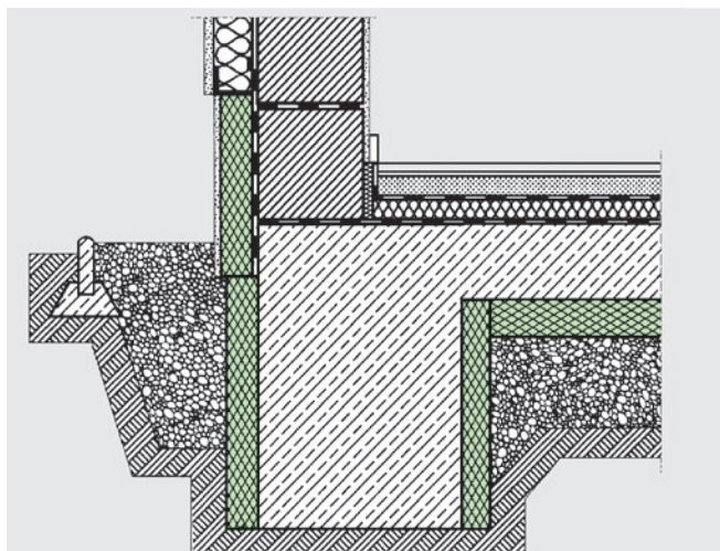
Afb. 19: Isolatie van de fundering en de aansluiting op het bovenliggende Isostuc systeem.
