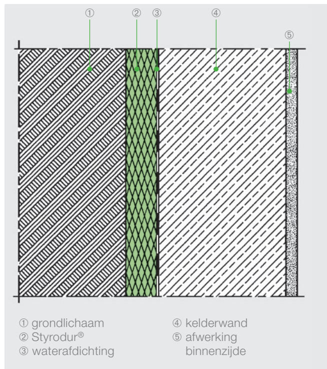
Afb. 1: Kelderwand met isolatie aan de buitenzijde.
