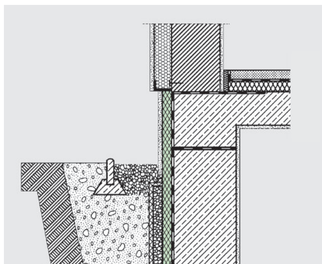
Afb. 10: Sokkelisolatie bij een Isostuc gevel.
