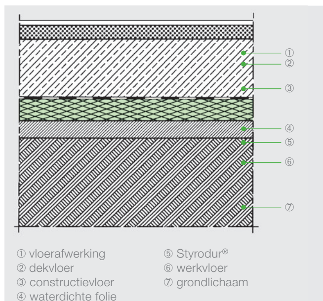
Afb. 2: Vloerisolatie zonder grondwater.
