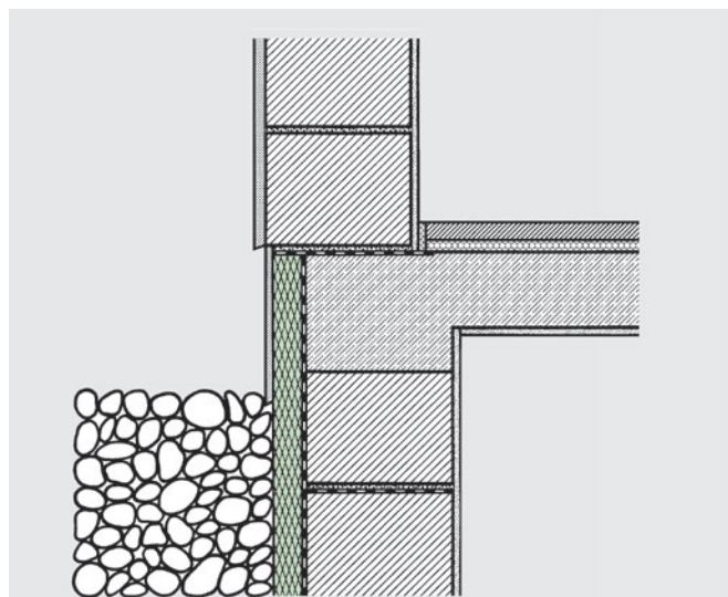
Afb. 9: Sokkelisolatie bij opgaand metselwerk.
