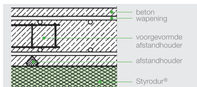
Afb. 17: Beloopbare onderste afstandhouder uit beton voor de onderwapening en een stalen afstandhouder voor de bovenwapening van de betonvloer
