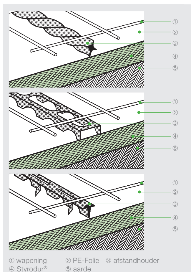
Afb. 18: Beloopbare kunststof afstandhouders voor wapeningsnetten. Door de verschillende profielhoogtes kan de juiste betondekking worden gekozen.
