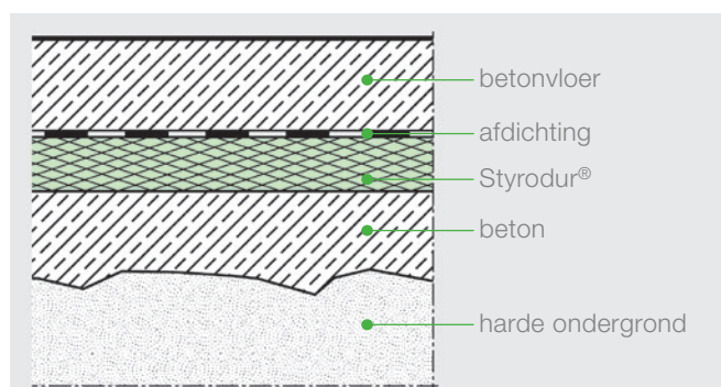
Afb. 15: Uitvlakken van de harde ondergrond met beton.
