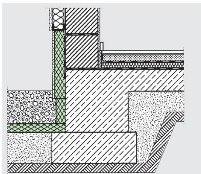
Afb. 20: Voorbeeld van een vorstschermb.
