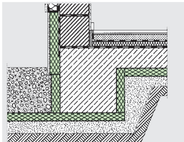
Afb. 21: Toepassing van Styrodur® platen onder dragende bouwdelen.
