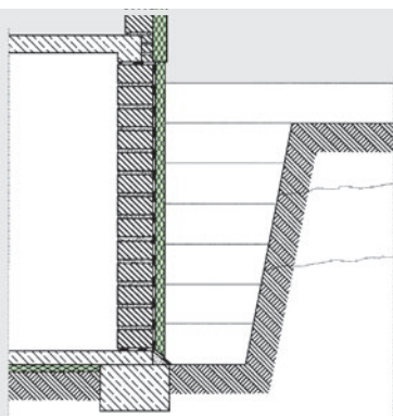
Afb. 24: Vullen in lagen en mechanisch verdichten van de grond.
