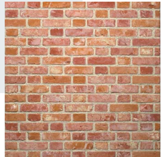
Tongerse Rijnvorm : Vlaams verband
