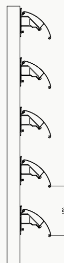
DucoSun 150 D verticaal
