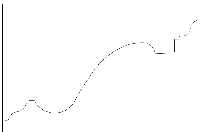
Doezastraat 2, 1632 Schaal: 1:5
