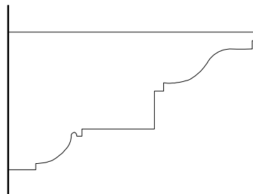
Aalmarkt 16, omstreeks 1580 Schaal: 1:5
