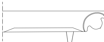
Hooigracht 67, tweede kwart 15de eeuw Schaal 1:5
