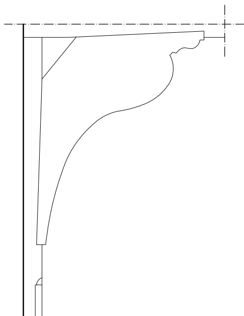
Mandemakersteeg 7, 1588 Schaal 1:5
