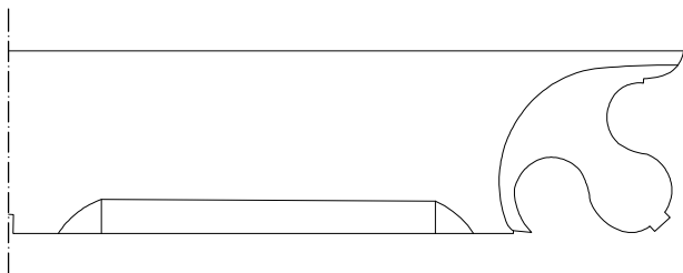
Breestraat 135, 1365 Schaal 1:5
