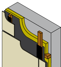
Houten draagconstructie
