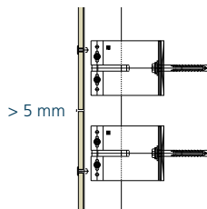
Aluminium draagconstructie met open horizontale voeg
