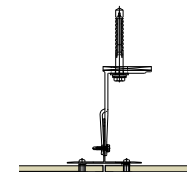
Aluminium draagconstructie, gesloten verticale voegoplossing
