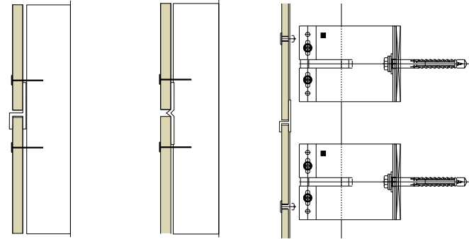
Houten draagconstructie met gesloten horizontale voeg
