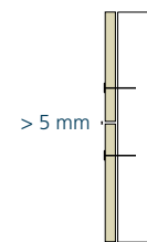
Houten draagconstructie met open horizontale voeg
