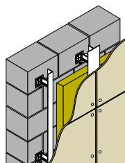
Aluminium draagconstructie
