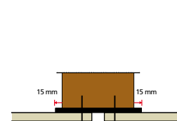
Houten draagconstructie, gesloten verticale voegoplossing
