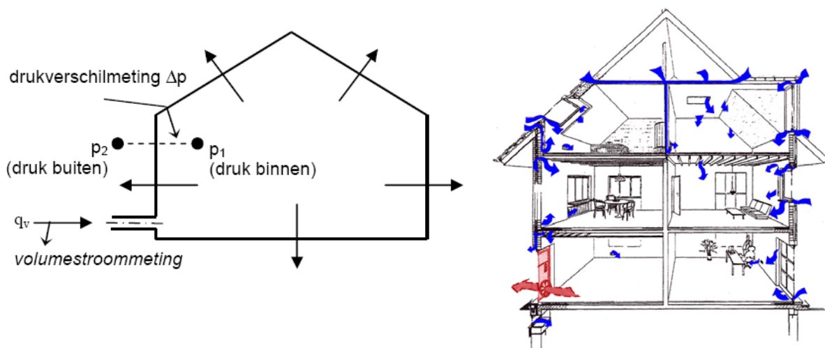
Principe luchtdoorlatendheidsmeting ( q_{v,10} -meting). Bron afbeelding 1: NEN en afbeelding 2: www.
