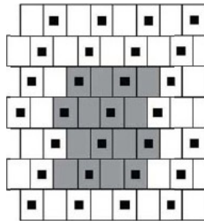
Dambordsgewijs verankeren in halfsteensverband
