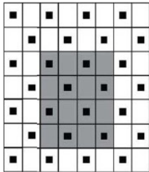
Dambordsgewijs verankeren van dakpannen
