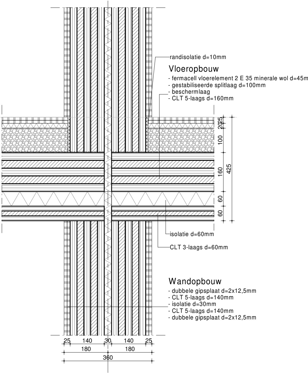
Woningscheidend detail bij modulair bouwen
