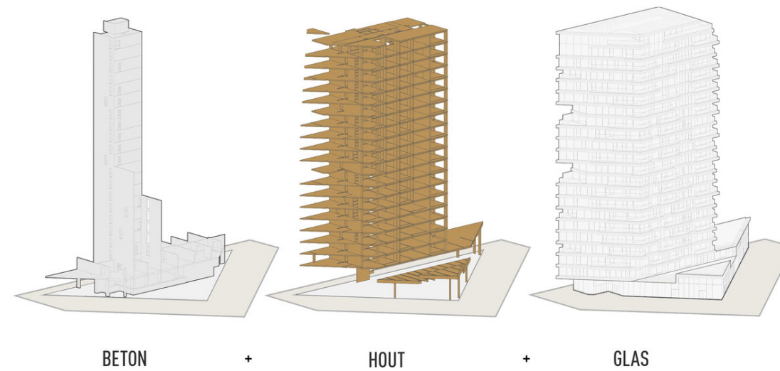
Constructiemodel HAUT - Team V Architectuur
