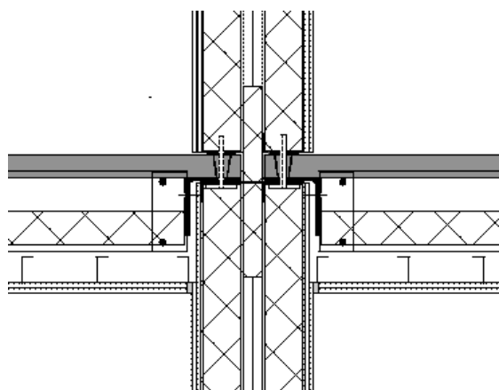
Voorbeelddetail woningscheidende knop
