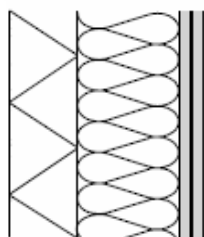
Voorbeeld opbouw Star-Frame wand
