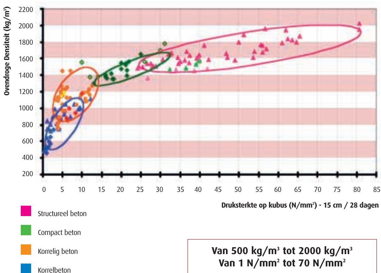
Correlatie tussen ovendroge dichtheid en druksterkte
